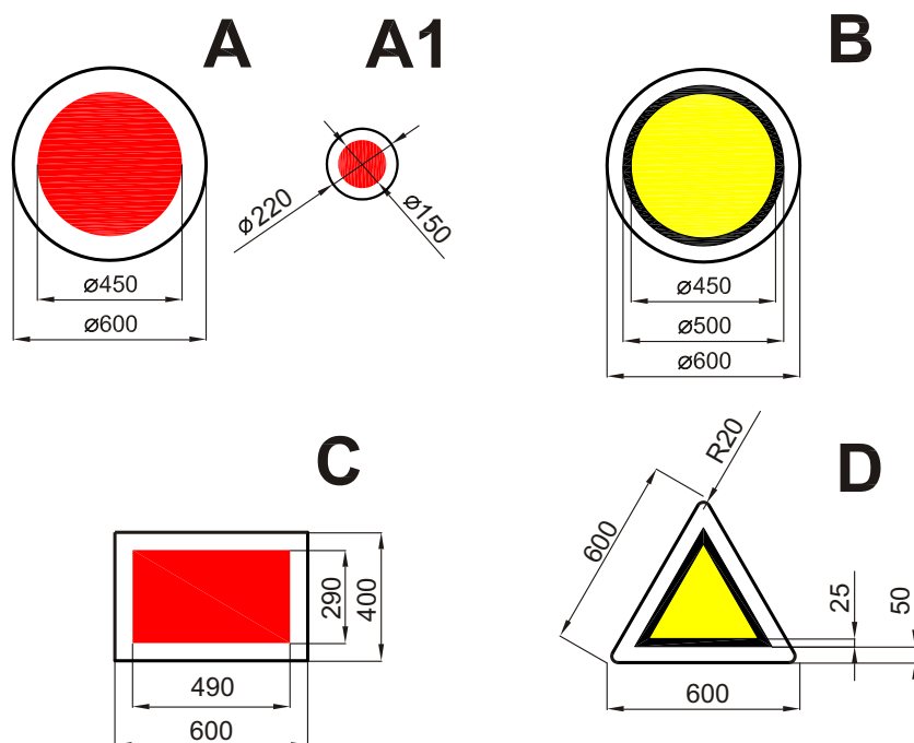
Obr. 43 Terče, desky a štíty přenosných návěstidel s návěstmi "Stůj" a "Výstraha"
