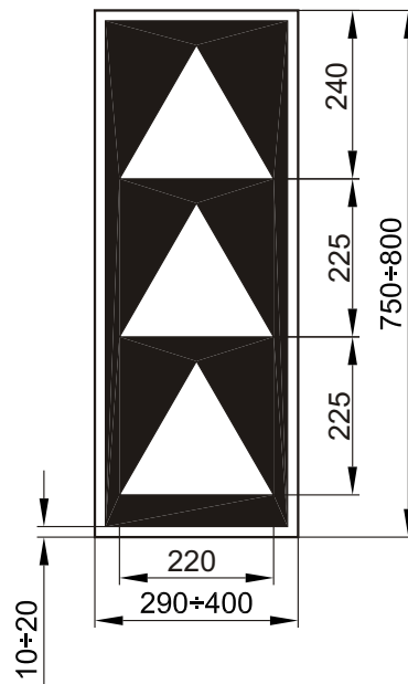
Obr. 18 Vzdálenostní upozorňovadla s návěstmi "Vlak se blíží k hlavnímu návěstidlu"
