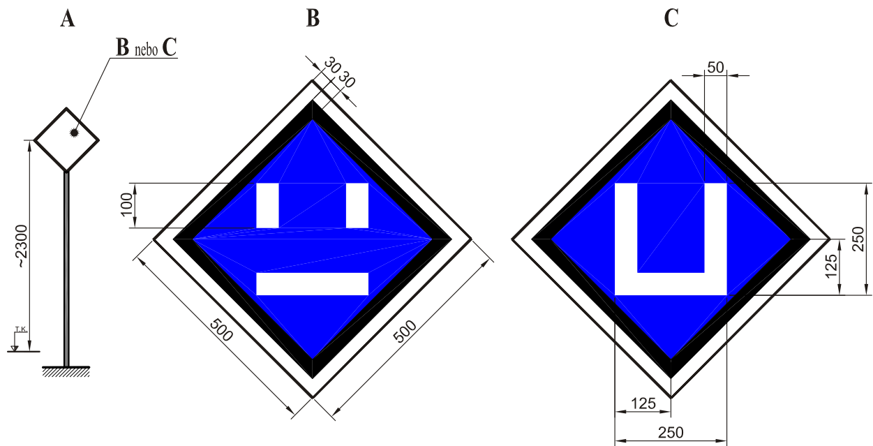
Obr. 41 Návěstidla pro obsluhu elektrického topení z motorových hnacích vozidel
