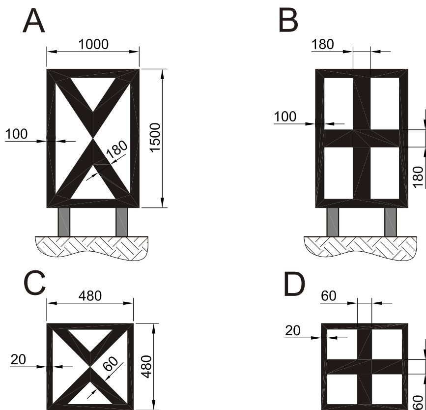
Obr. 13 Předvěstní upozorňovadla s návěstmi "Stanoviště samostatné předvěsti"
