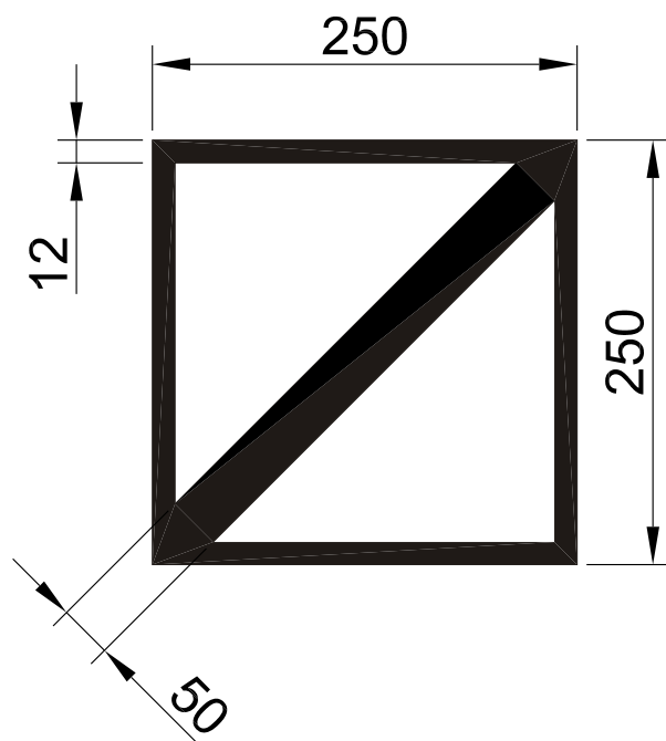
Obr. 11 Návěstní upozorňovadlo s návěstí "Skupinové návěstidlo"
