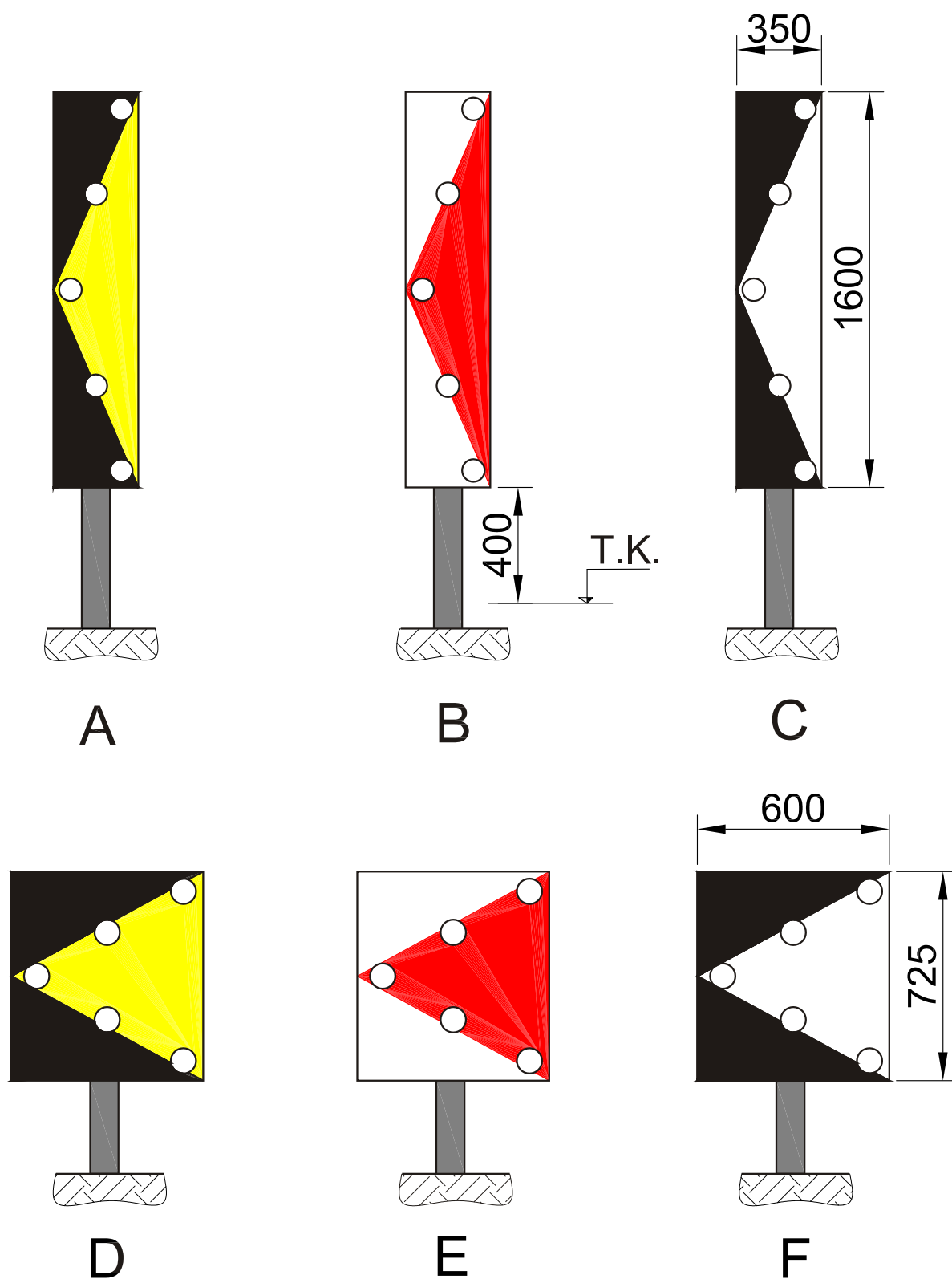
Obr. 12 Návěstní upozorňovadla s návěstmi "Hlavní návěstidlo je na opačné straně", "Samostatná předvěst je na opačné straně", "Přejezdník je na opačné straně"
