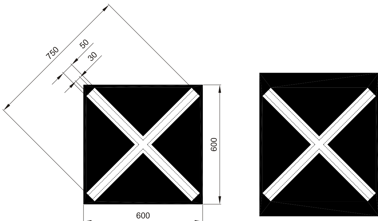
Obr. 41 Návěstidla pro obsluhu elektrického topení z motorových hnacích vozidel
