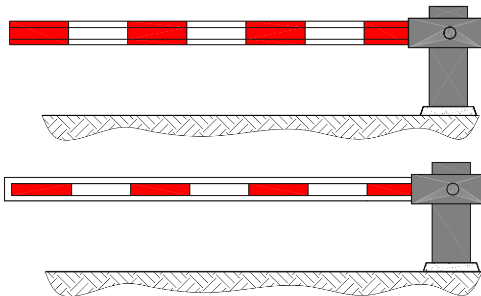
Obr. 35 Příklady provedení nátěrů závory s odrazným pásem
