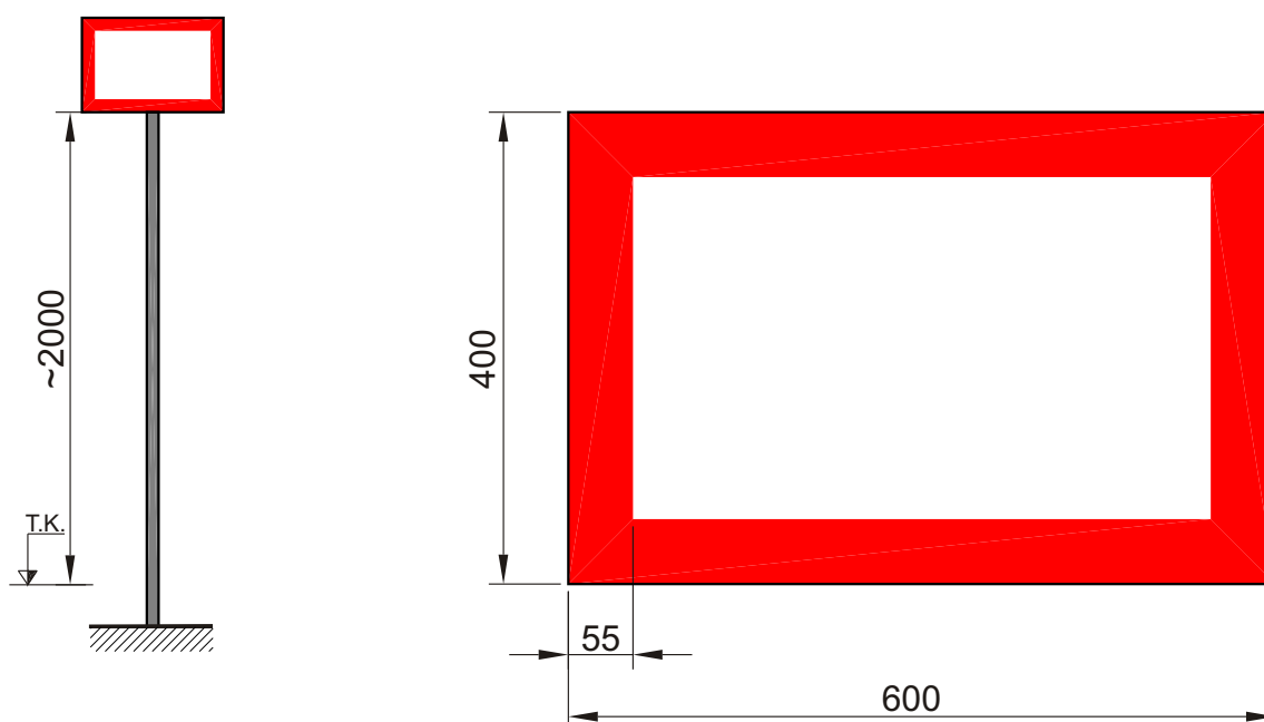
Obr. 40 Návěstidlo s návěstí "Místo zastavení"
