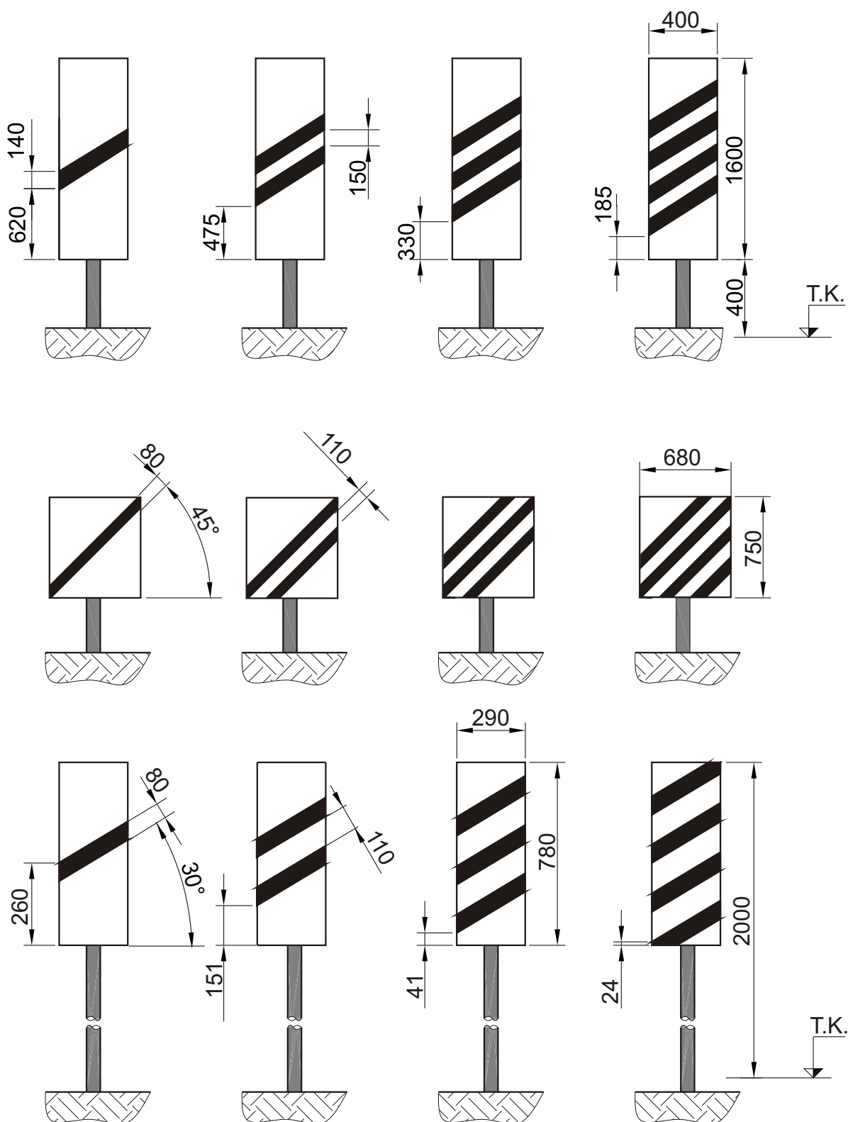
Obr. 15 Vzdálenostní upozorňovadla s návěstí "Vlak se blíží k samostatné předvěsti" před předvěst vjezdového, cestového nebo odjezdového návěstidla a před tabulku s křížem, která takovou předvěst nahrazuje
