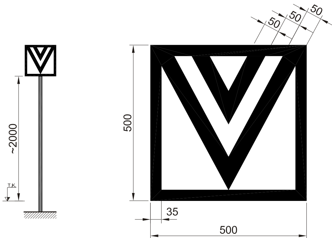
Obr. 39 Návěstidlo s návěstí "Hranice pro návrat vozidel z širé trati"
