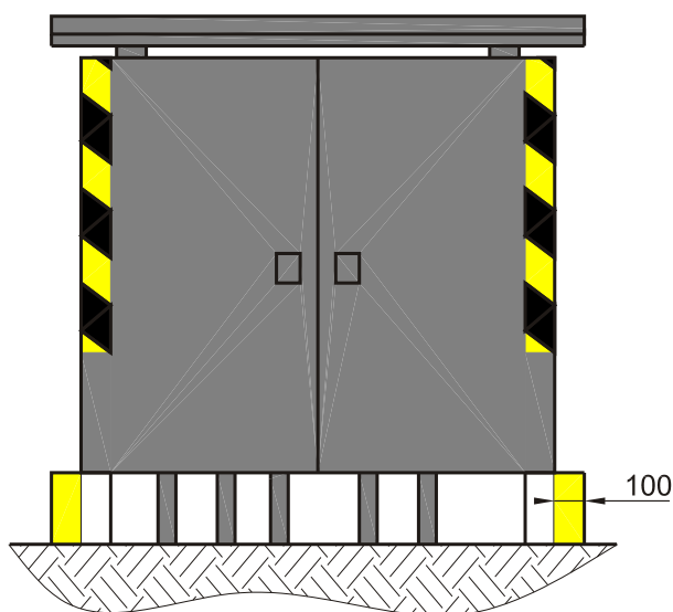
Obr. 59 Reléová skříň
