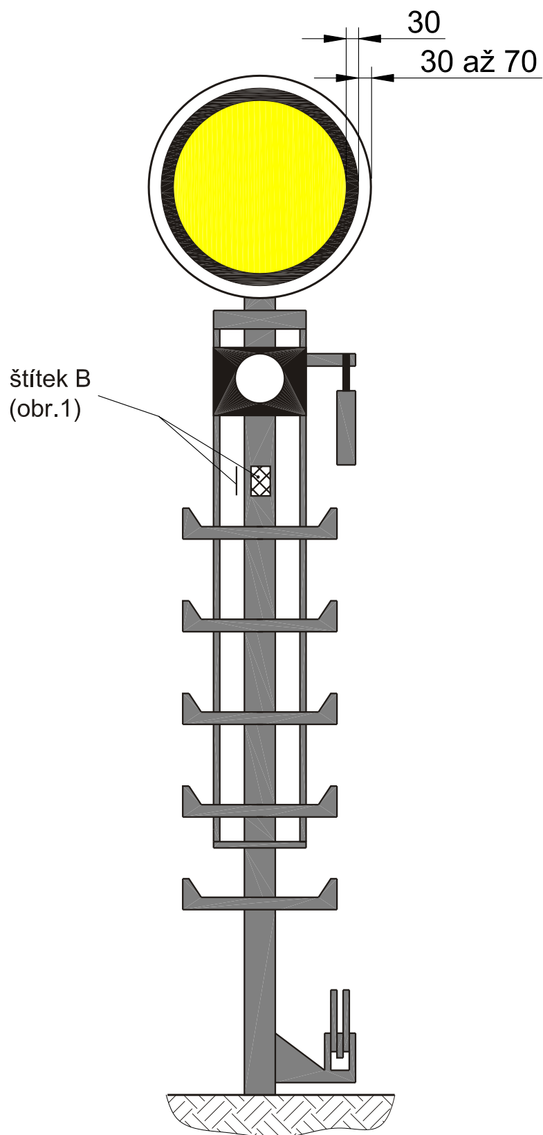
Obr. 6 Mechanická dvouznamková předvěst
