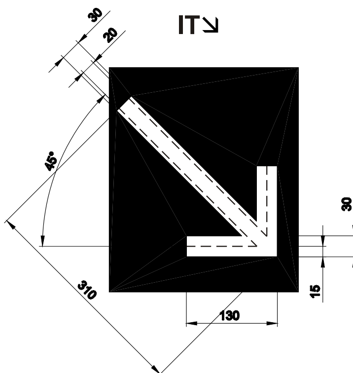
Obr. 3 Indikátorové tabulky
