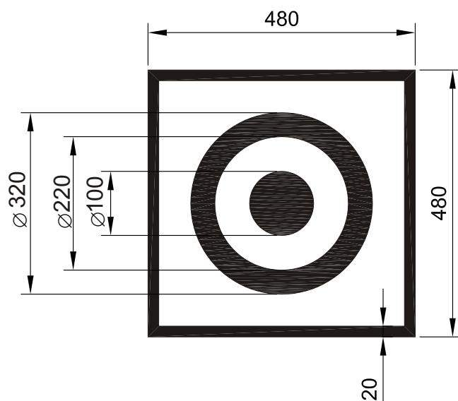
Obr. 14 Předvěstní upozorňovadlo s návěstí "Stanoviště oddílového návěstidla"
