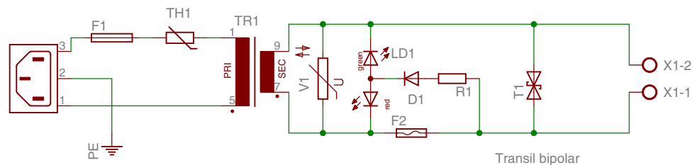
Zdroj střídavého proudu pro DCC booster s jistěním
