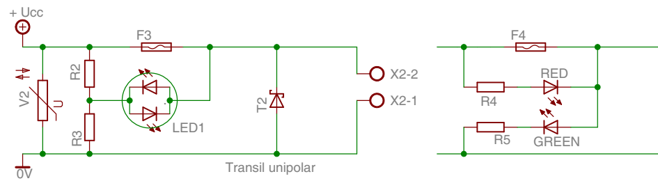
Jistění pro zdroj stejnosměrného proudu
